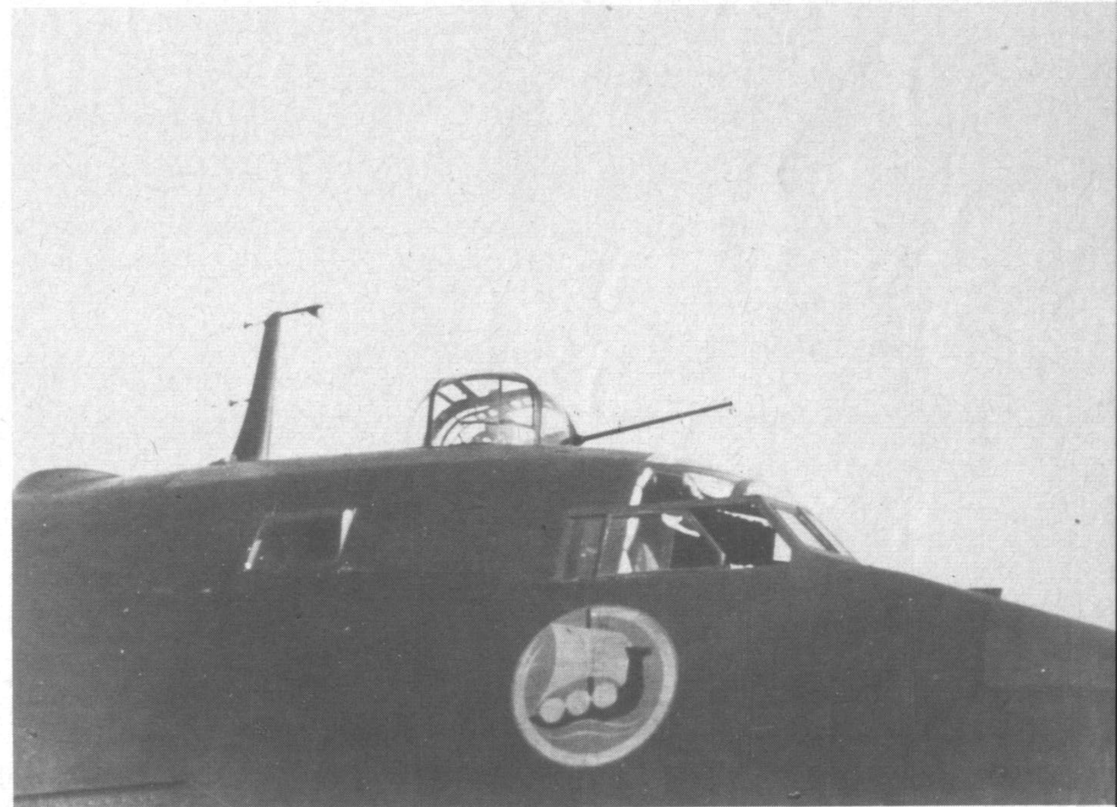
Drehturm mit MG 151 hinter dem Führerraum der Bv 222 V 4. Staffelabzeichen der LTS 222 gut sichtbar.
